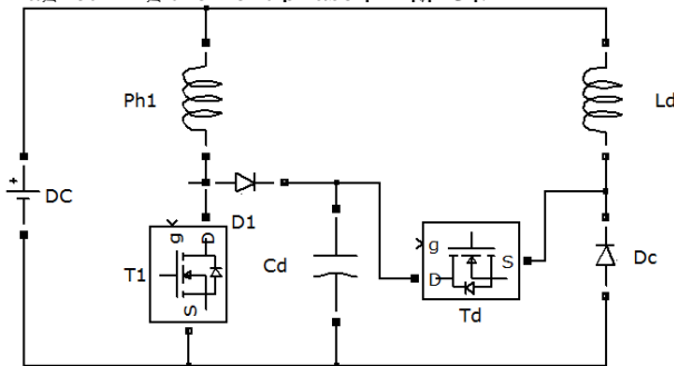
Fig. 3. C-Dump converter
