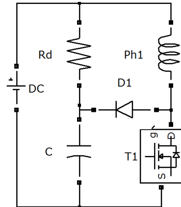
Fig. 5. R-dump converter
