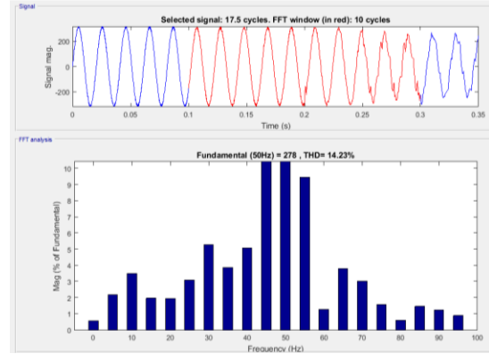
(b) PSO
