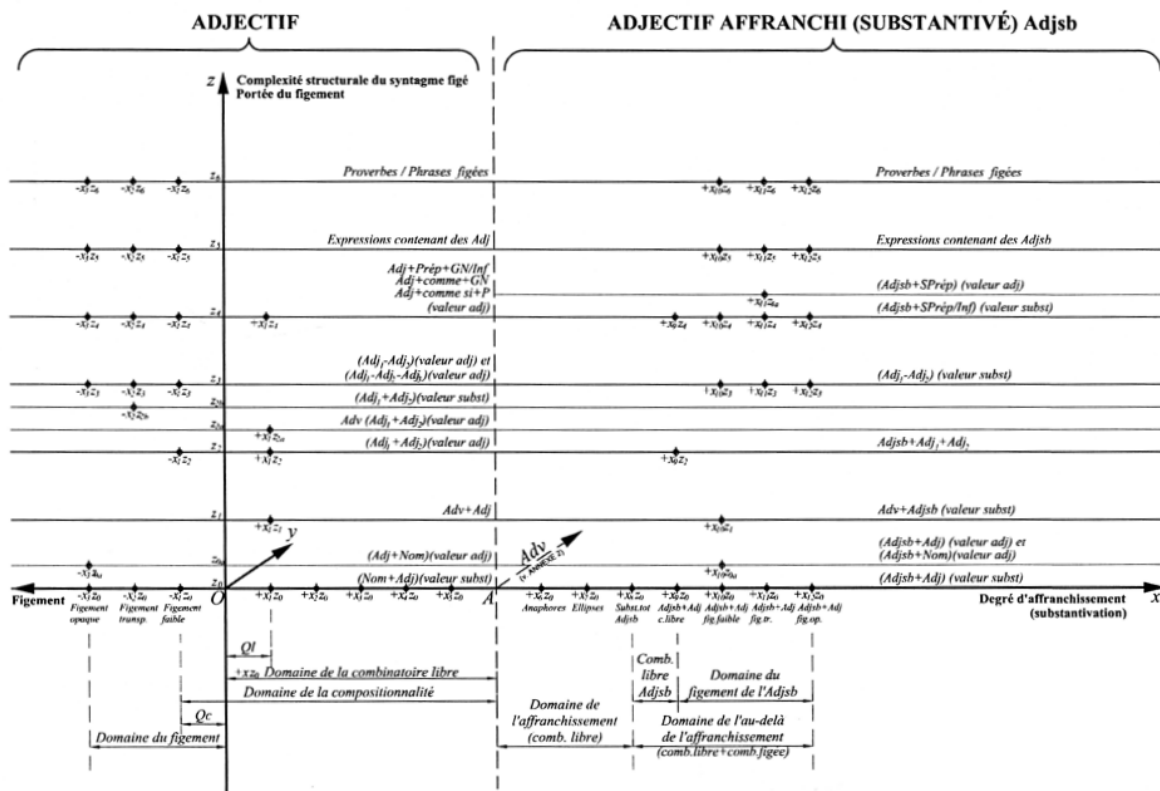
SCHÉMA DU MODÈLE MATHÉMATIQUE TRIDIMENSIONNEL - SUBSTANTIVATION
