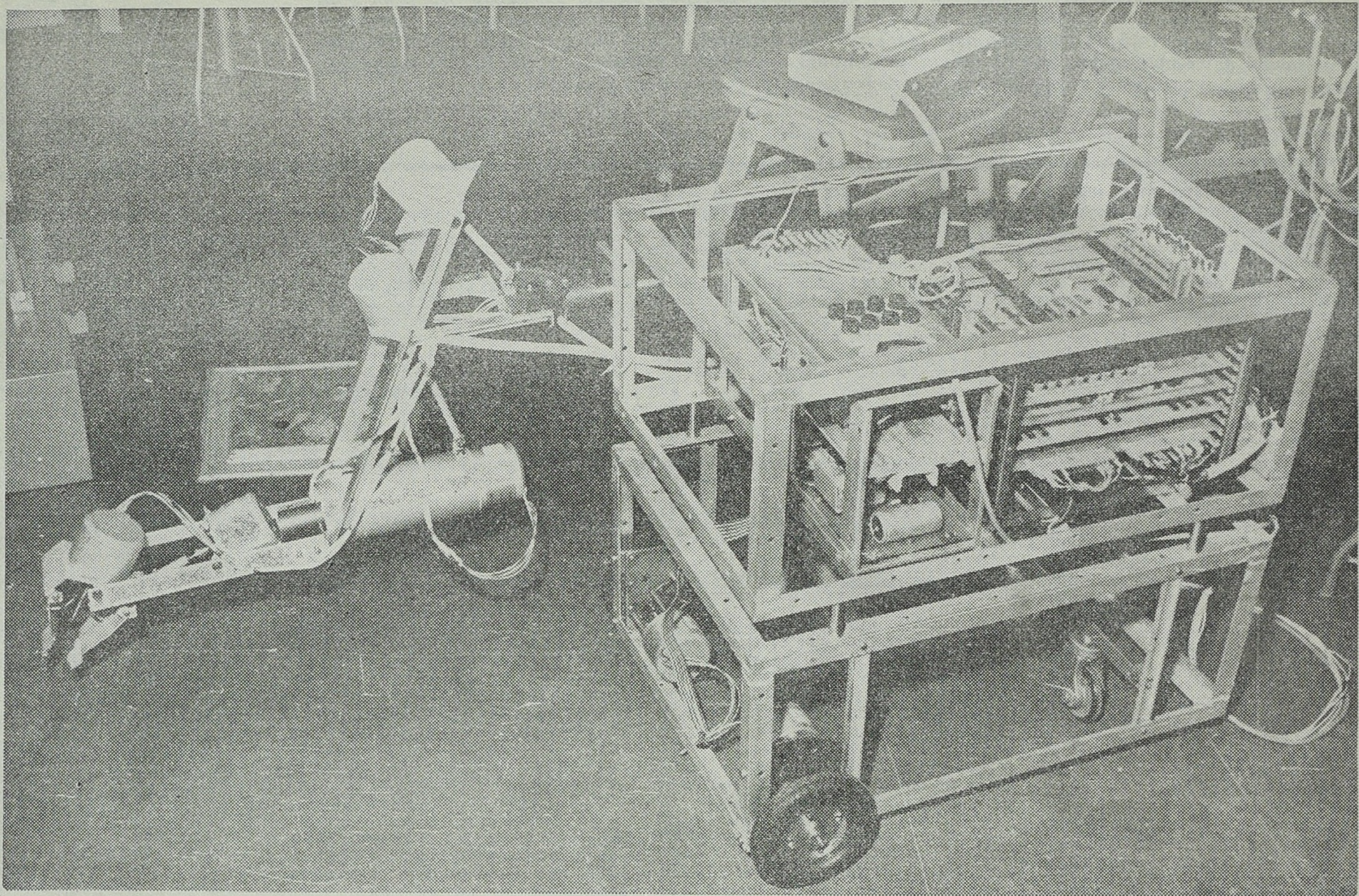
Robotul experimental din imagine — un complicat și modern sistem mecatronic — se află în stadiul ultimelor încercări. El înglobează rezultatele mai multor proiecte de diplomă elaborate de studenți ai facultăților de Mecanică și Electrotehnică.
