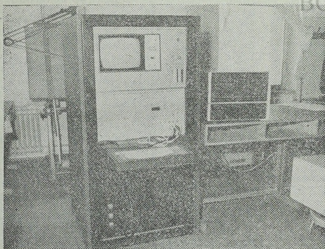
Sistem pentru testarea plachetelor echipate din tehnologia P a calculatorului Felix C-256 în cadrul căruia stimulii de test sint memorați, iar evaluarea răspunsurilor în vederea detecției se realizează prin comparare.
