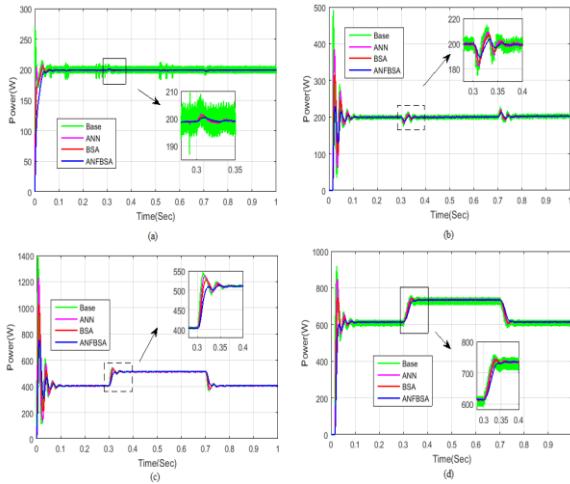
Fig. 6. Comparison analysis of (a) PV (b) Wind (c) Battery (d) Load
