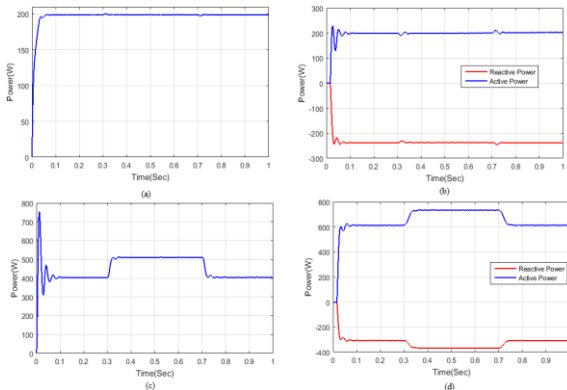
Fig. 5. Performance analysis of (a) PV (b) Wind (c) Battery (d) Load
